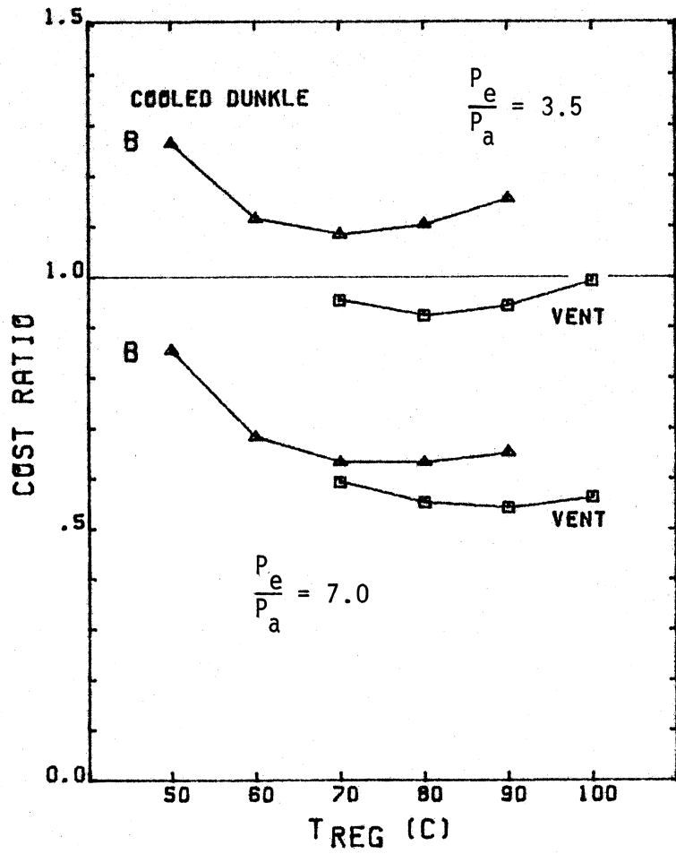
Figure 6.4.1 (cont) Miami, gas-fired. (c) & (d) cost ratios.
