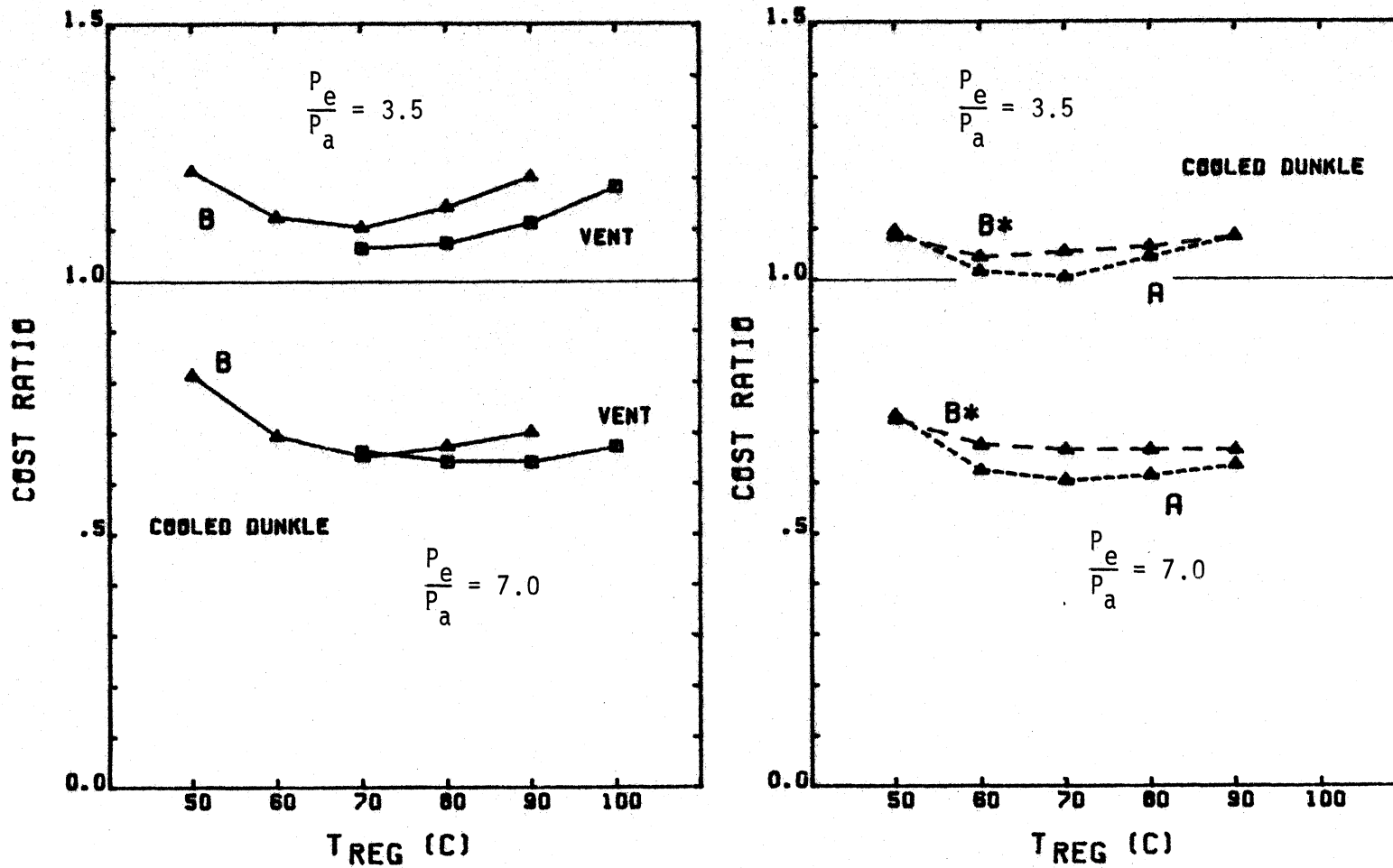
Figure 6.4.6 (cont) Columbia, gas-fired. (c) & (d) cost ratios.
