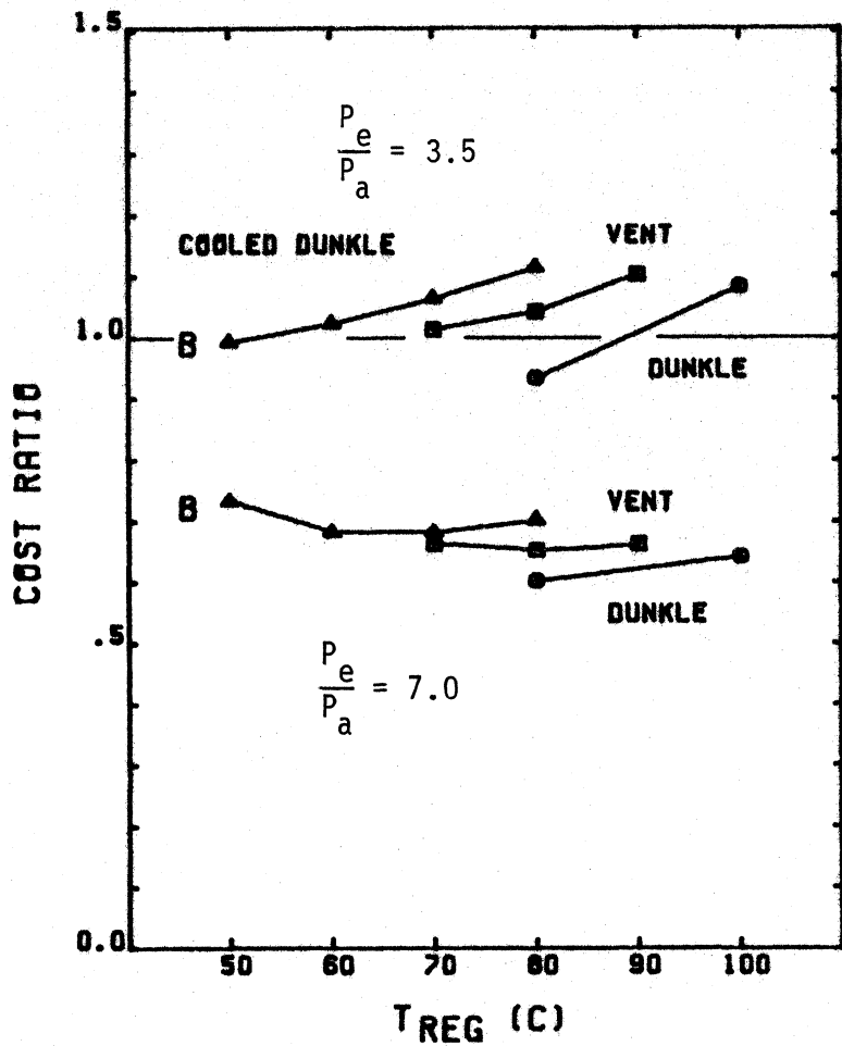
Figure 6.4.4 (cont) Phoenix, gas-fired. (c) & (d) cost ratios.
