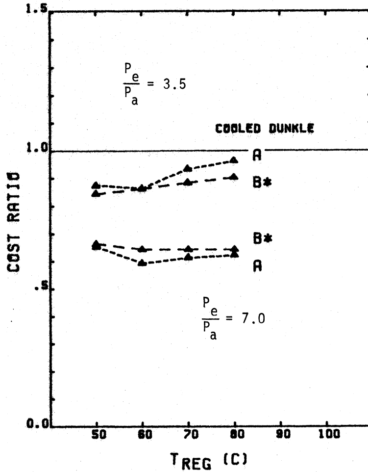
Figure 6.4.4 (cont) Phoenix, gas-fired. (c) & (d) cost ratios.
