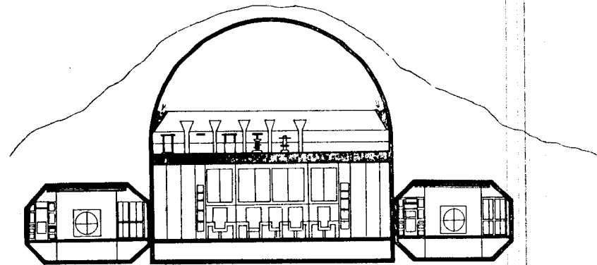
SECTION D-D
