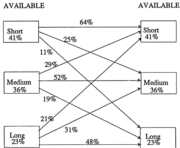
Figure 7. Conditional Probability of AV to AV State Changes
